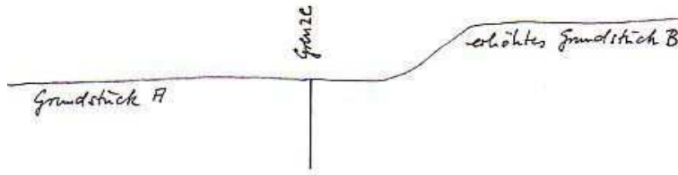
Abb. 5 Zulässige unbefestigte Erhöhung mit Böschung und Abstandsfläche
